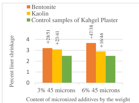
شکل 8. نمودار تغییرات درصد انقباض خطی کاهگل تهیه شده با مواد افزودنی 45 میکرون در مقایسه با کاهگل معمولی Fig.8. Variation of percent of linear shrinkage of modified samples of Kahgel plaster with additives 45 microns
