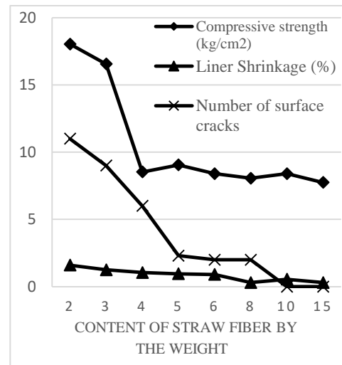
شکل 2. نتایج آزمایش ژئوتکنیک نمونه‌های مختلف اندود کاهگل با درصدهای متفاوت الیاف کاه
