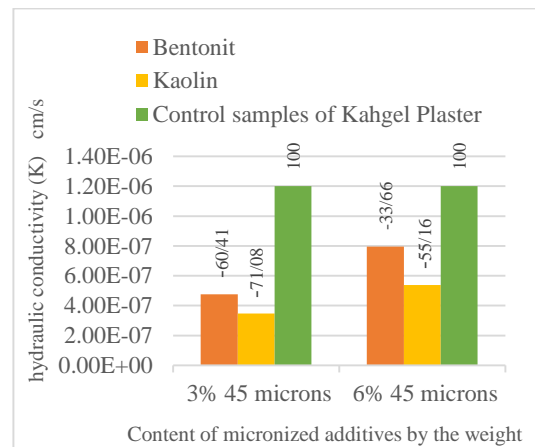
شکل 4. نمودار تغییرات ضریب نفوذپذیری کاهگل تهیه شده با مواد افزودنی 45 میکرون در مقایسه با کاهگل معمولی
