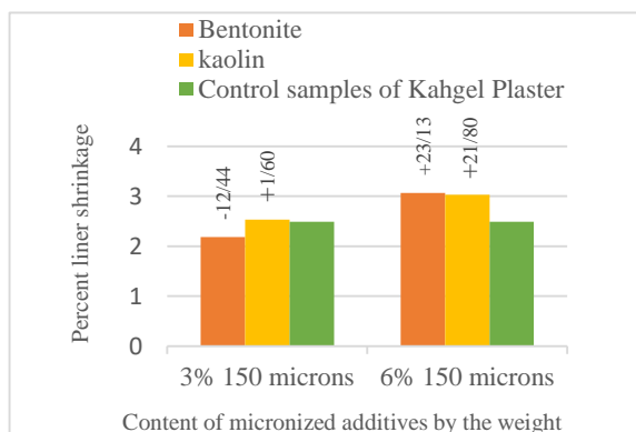
شکل 7. نمودار تغییرات درصد انقباض خطی کاهگل تهیه شده با مواد افزودنی 150 میکرون در مقایسه با کاهگل معمولی Fig.7. Variation of percent of linear shrinkage of modified samples of Kahgel plaster with additives 150 microns
