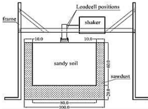
شکل ۲: نمای جانبی مدل فیزیکی برای حالت پی بدون عمق مدفون (اندازه‌ها به سانتی متر هستند).
