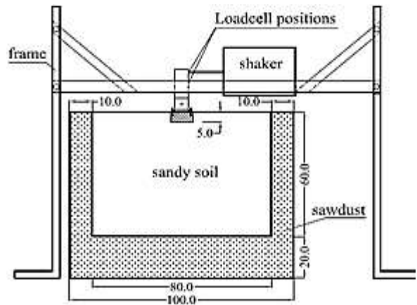
شکل ۴: نمای جانبی مدل فیزیکی برای حالت پی کاملاً مدفون (اندازه‌ها به سانتی متر هستند).
