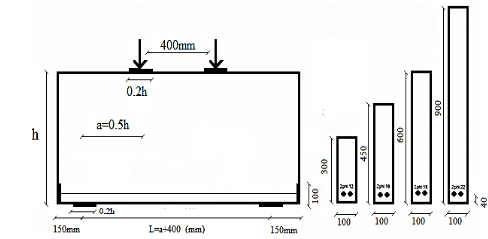
شکل ۳: هندسه نمونه‌ها
