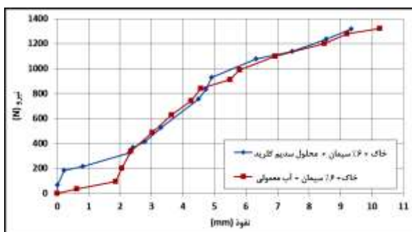
شکل ۵: نتایج آزمایش CBR بر روی خاک + ۶٪ سیمان همراه با آب معمولی و محلول سدیم کلرید
