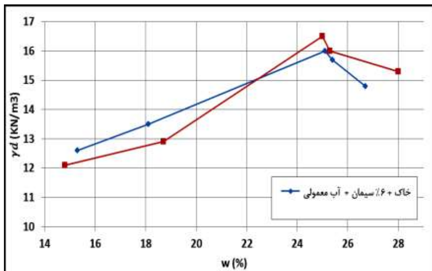
شکل ۸: نتایج آزمایش تراکم بر روی خاک اولیه + ۶٪ سیمان + آب + محلول سدیم کلرید
