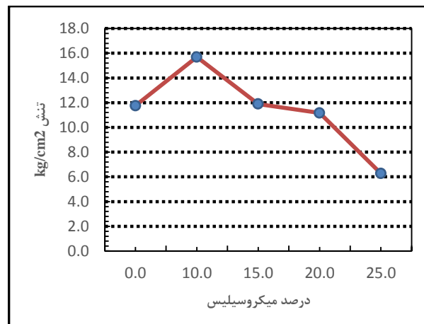
شکل ۴: تنش تک محوره برای دوره زمانی ۷ روز
