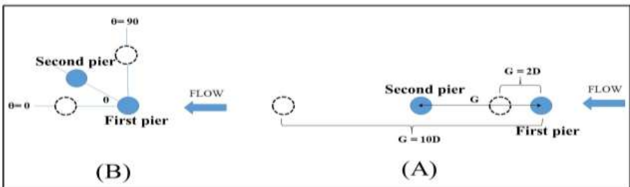
شکل ۲. چیدمان پايه ها برای (A) تغییرات طولی فاصله بين پايه ها و (B) تغییرات زاويه ای
