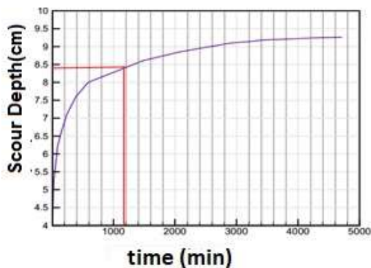
شکل ۳. نمودار پیشرفت عمق آبستگي بر حسب زمان برای پايه جلویی در آزمون بلند مدت
