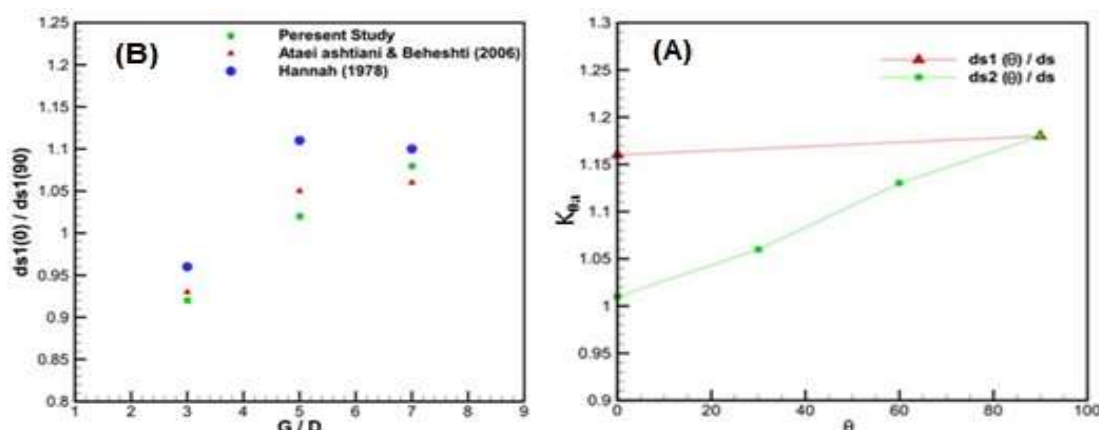
شکل 6. نتایج آزمایشات مربوط به گروه پایه‌ها تحت زاویه نسبت به راستای جریان (A) تغییرات نسبت عمق آبشستگی در پایه اول و دوم تحت زاویه به عمق آبشستگی تک پایه در زوایای مختلف در شرایط G=3D (B) مقایسه نتایج پژوهش حاضر با مطالعات محققین قبل
