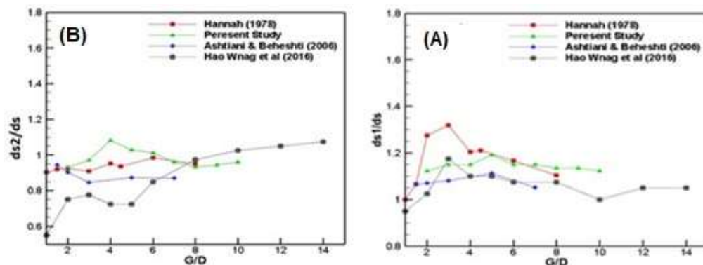
شکل 5. مقایسه نتایج آزمایشات فعلی با نتایج محققین پیشین در چیدمان دو پایه در راستای جریان. (A) برای پایه اول. (B) برای پایه دوم Fig. 5. Comparison between present study and previous scholars in 2-pier layout (A) First pier (B) Second pier
