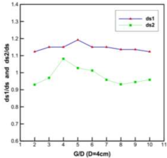
شکل 4. تغییرات عمق حفرة آبستگي در پایه اول و دوم نسبت به آبستگي تک پایه در مقابل تغییرات فاصله بین پایه‌ها
