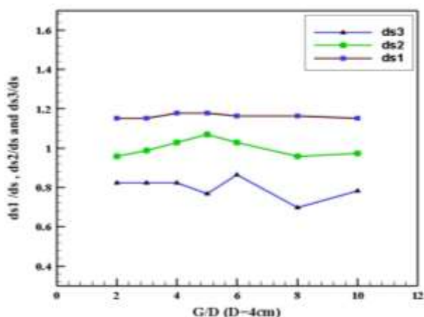
شکل 7. تغییرات عمق حفره آبستگي در پایه اول، دوم و سوم نسبت به آبستگي تک پایه در مقابل تغییرات فاصله بين پایه ها Fig. 7. Scour depth variation for first, second and third pier with pier space variation
