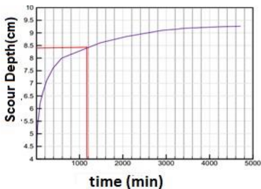
شکل 3. نمودار پیشرفت عمق آبستگي بر حسب زمان برای پايه جلویی در آزمون بلند مدت
