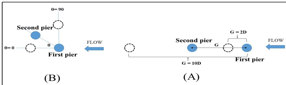
شکل 2. چیدمان پايه ها برای (A) تغییرات طولی فاصله بین پايه ها و (B) تغییرات زاویه ای
