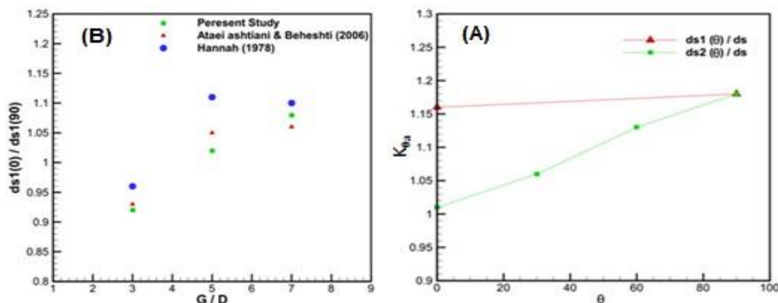
شكل 6. نتايج آزمايشات مربوط به گروه پايه‌ها تحت زاويه نسبت به راستاي جريان (A) تغييرات نسبت عمق آبستگي در پايه اول و دوم تحت زاويه به عمق آبستگي تك پايه در زواياي مختلف در شرايط G=3D (B) مقايسه نتايج پژوهش حاضر با مطالعات محققين قبل Fig. 6. Experimental results for angular pier group (A):The Ratio of Scour depth at first and second pier in angular pier group to single pier in G = 3D (B): comparison between results of present study and Previous scholars
