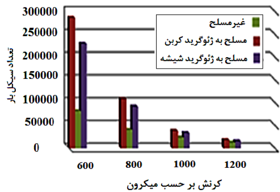
شکل ۴: نمودار میله‌ای (عمر نمونه‌ها - کرنش)
