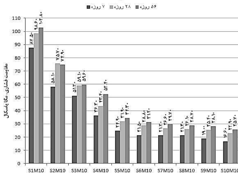
شکل ۳: مقاومت فشاری نمونه‌های حاوی ۱۰ درصد میکروسیلیس
