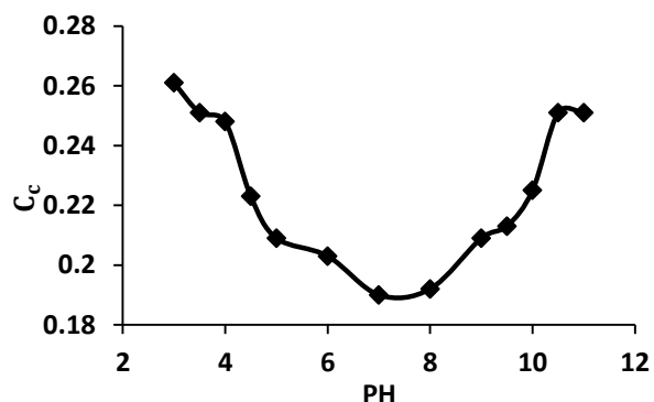
شکل ۶- تغییرات شاخص تراکم پذیری بر حسب تغییرات pH
